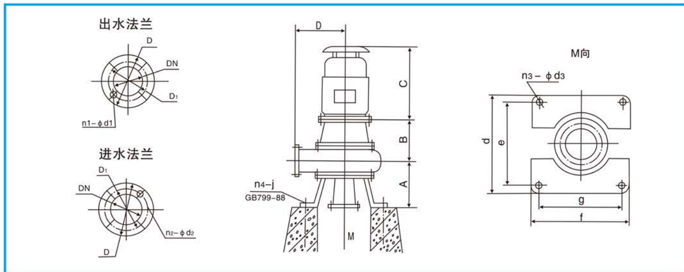
《《《 LW型泵外形及安装尺寸表 《《《
