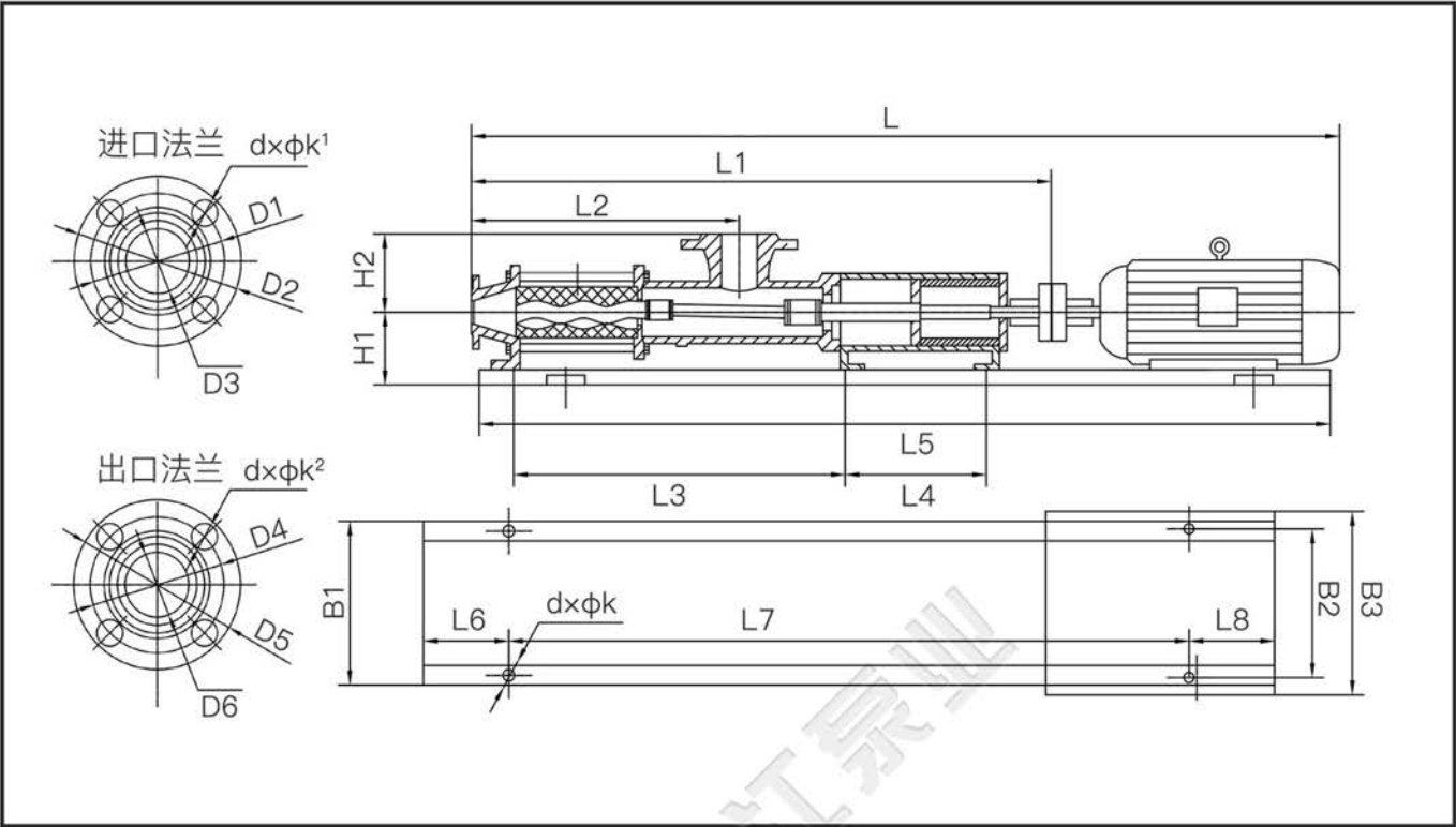
泵的安装尺寸 ( 固定转速时的尺寸，特定转速的安装尺寸在订货时附给)
