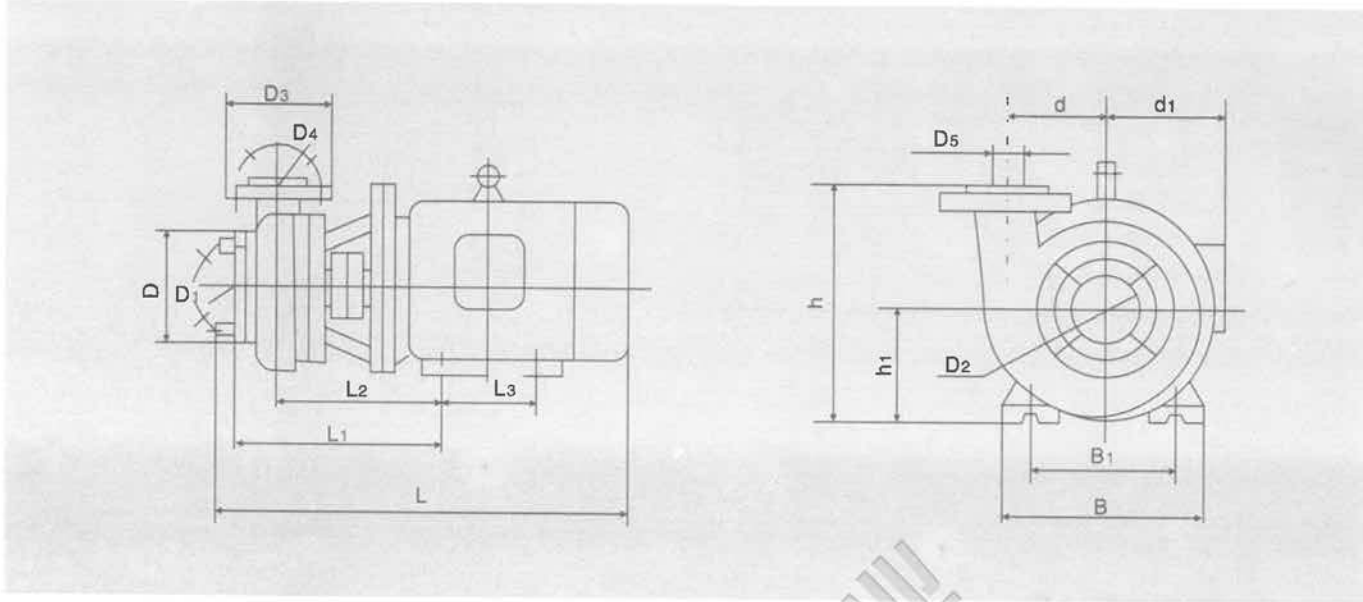
FSB-D短支架式安装示意图
